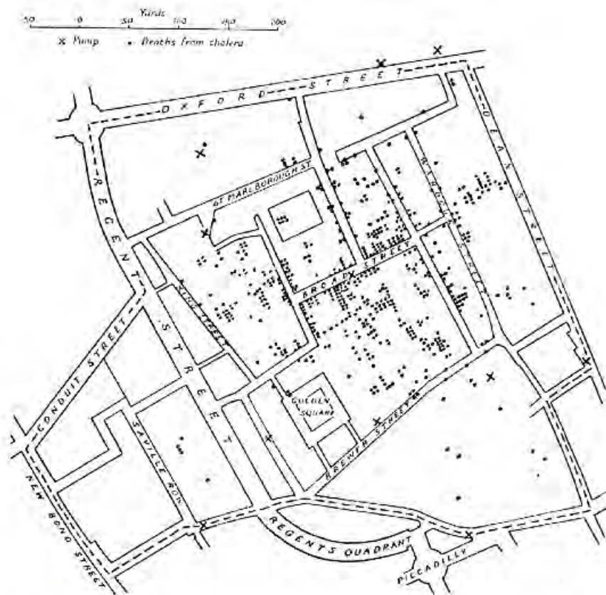
Mapa del Dr. Snow. Los puntos son casos de cólera y la cruces X los pozos de agua de donde bebía la población. El pozo de Broad Street era el contaminado, donde se agrupan más los casos. Fuente: Wikipedia.
