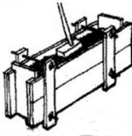
Tapia, diagrama reproducido de Mud por Laurie Baker. Nótese la formaleta y el pisón de madera.
