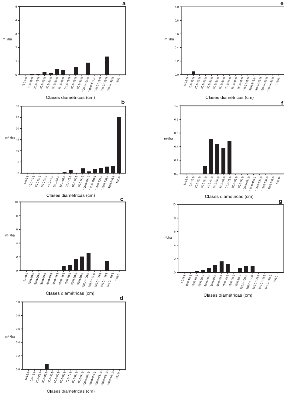
Figura 9. Distribución de área basal en especies demasiado escasas para caracterizar sus distribuciones diamétricas. a) C. odorata , b) C.pentandra , c) Fabaceae sp. , d) Dussia sp. , e) P. guatemalensis , f) P. dimorphandrum , g) S. macrophylla .. Escalas diferentes entre figuras.
