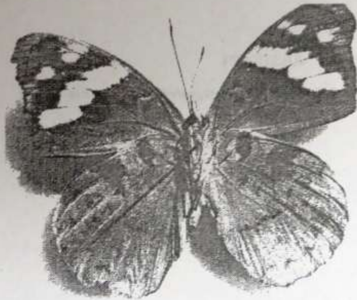
Fotos de Eunica mygdonia , dorsal (arriba) y ventral (abajo).
