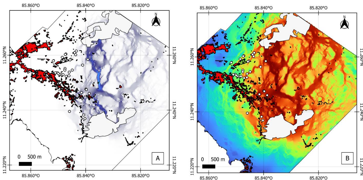
Figura 6. Conectividad resultante de las resistencias entre los tipos de suelo, A) en color azul es la distancia más corta y la menor resistencia encontrada, B) Se marcan en coloración roja los todos los circuitos encontrados, mayor coloración mayor probabilidad de desplazamiento.
