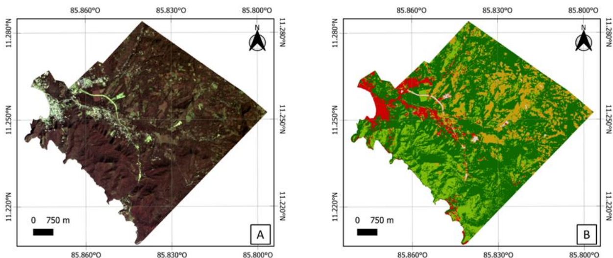
Figura 2. Generación de imágenes por clasificación supervisada, con 87.8% de precisión general A) se observa el ráster virtual con las bandas R:2 G:1 B:3, B) clasificación generada y limpia a partir del plugin Dsetzaka .
