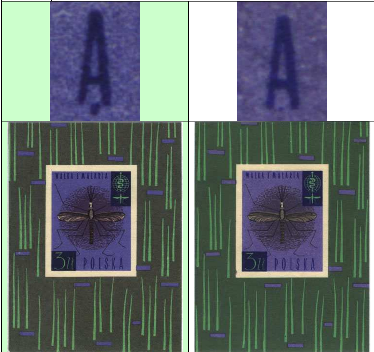
Diptera : Culicidae.
