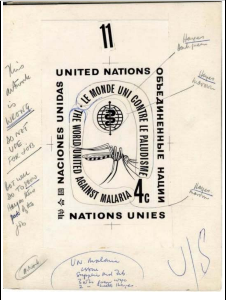
Diptera : Culicidae
