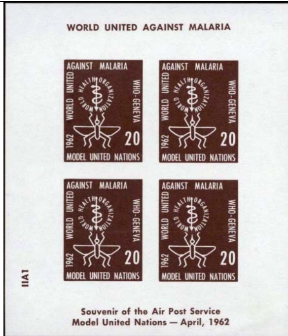
Lámina IIA1
