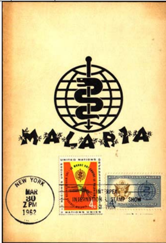
Diptera : Culicidae
