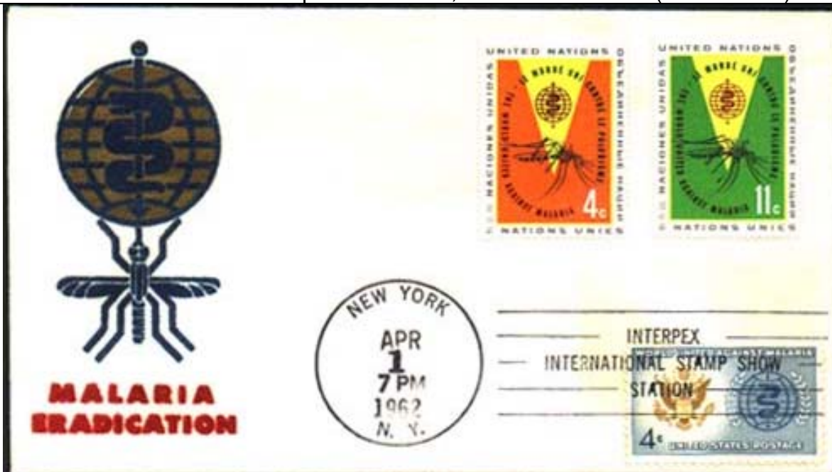
Diptera : Culicidae
