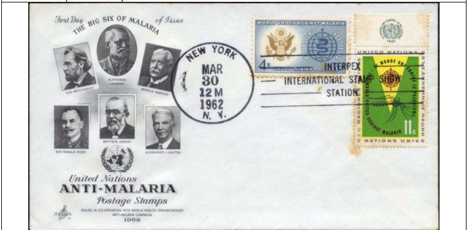
Diptera : Culicidae
