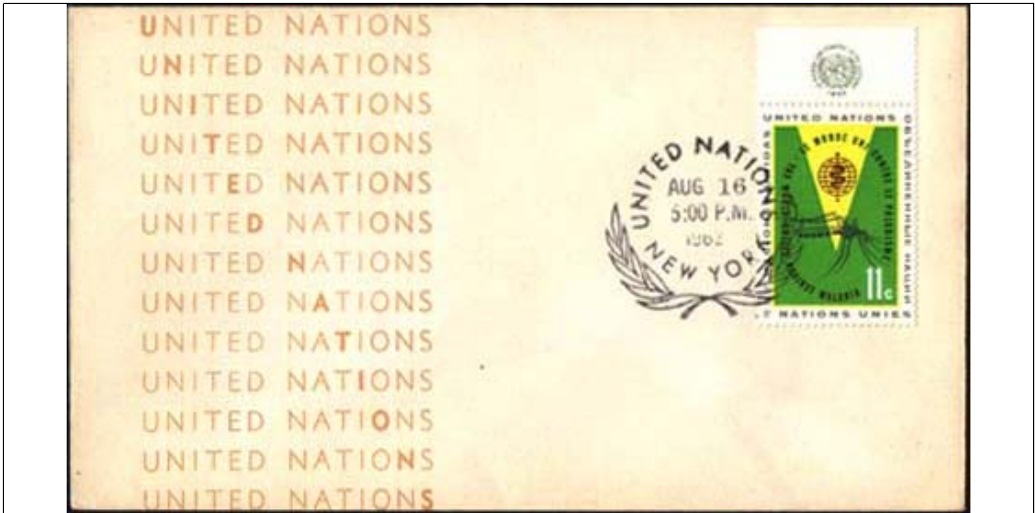
Diptera : Culicidae
