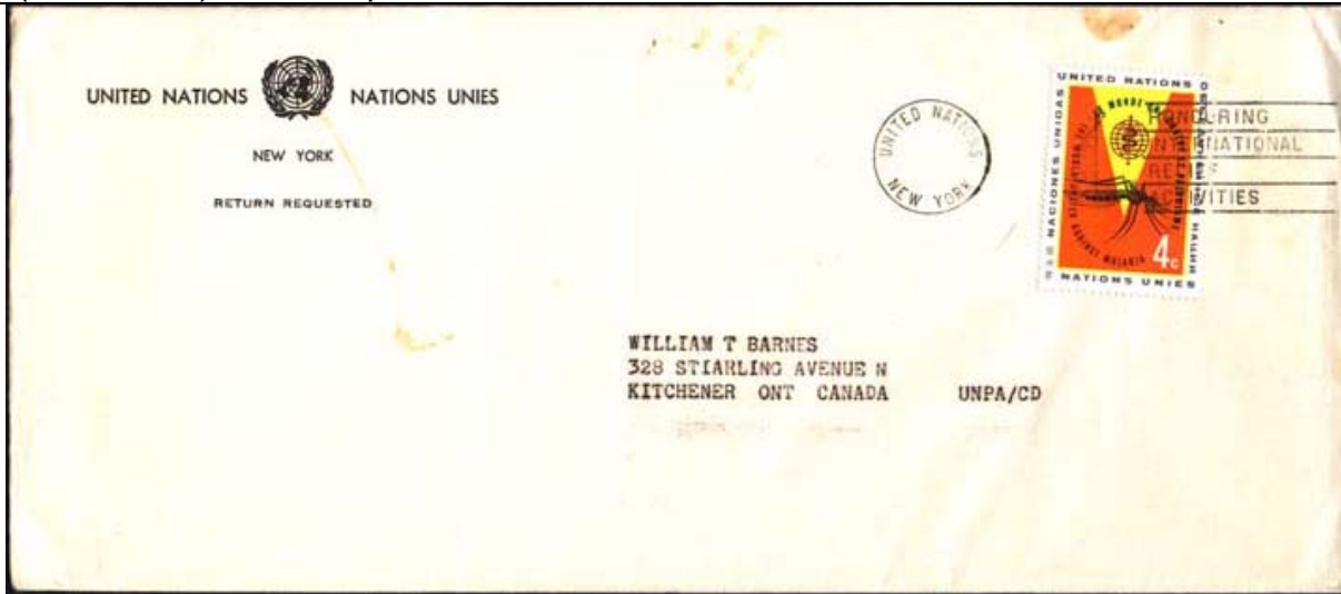
Diptera : Culicidae
