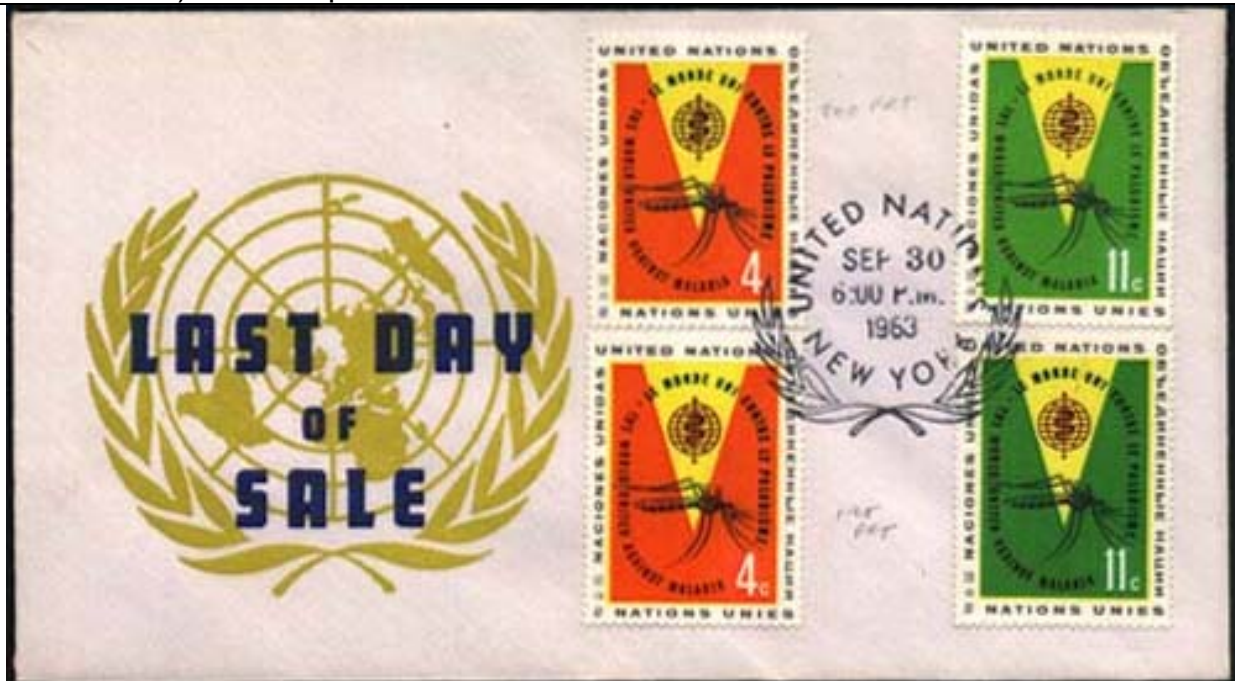
Diptera : Culicidae
