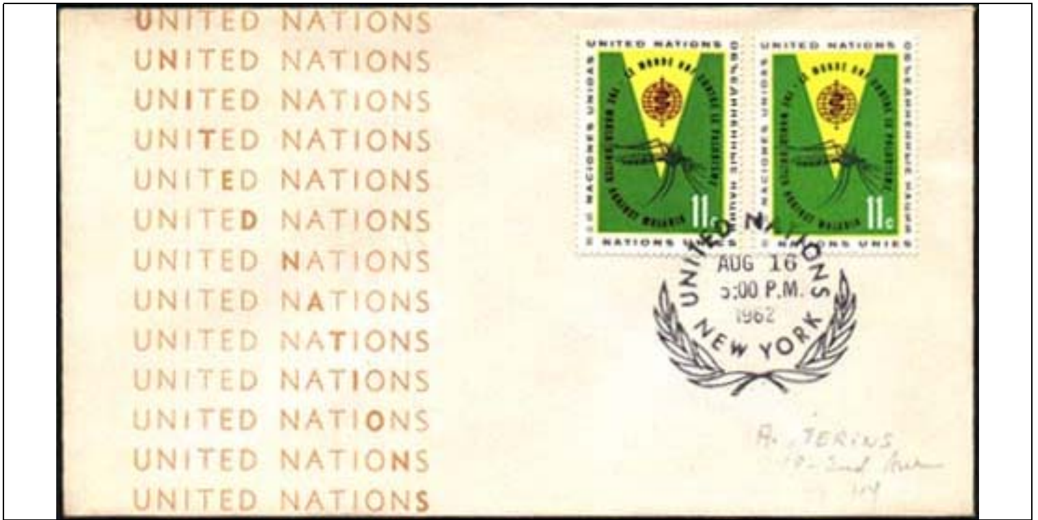
Diptera : Culicidae
