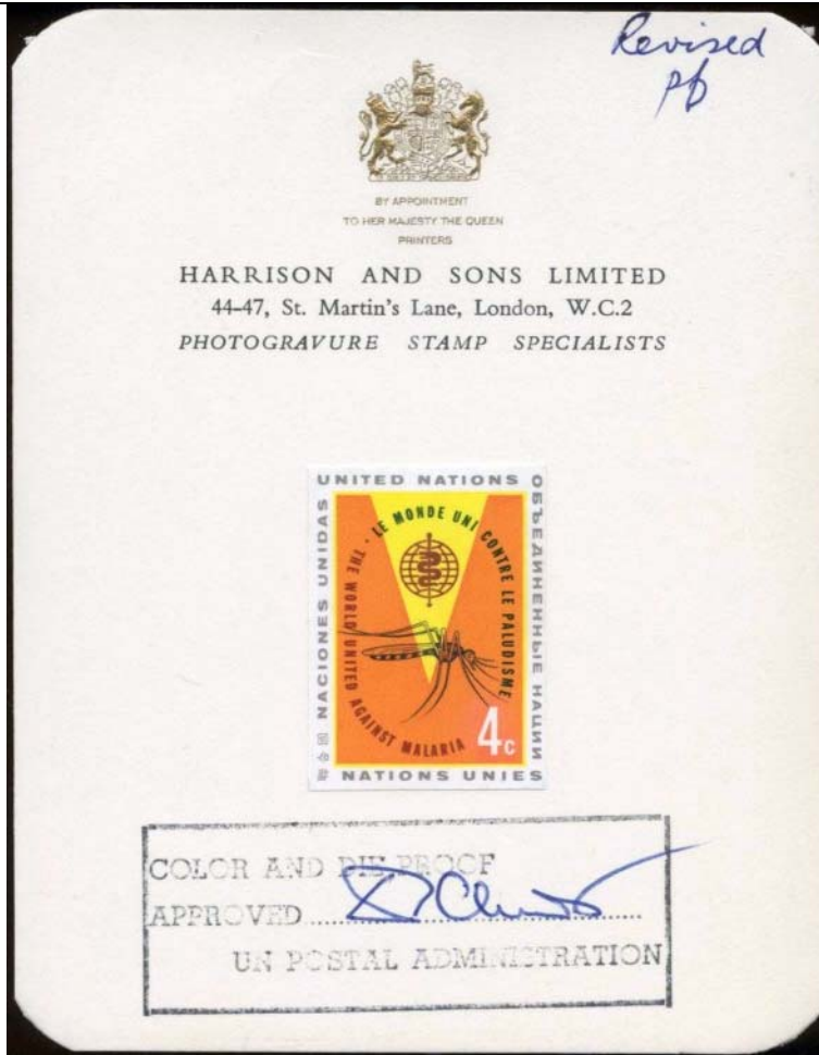
Diptera : Culicidae
