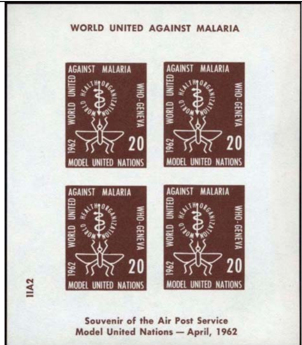
Lámina IIA2
