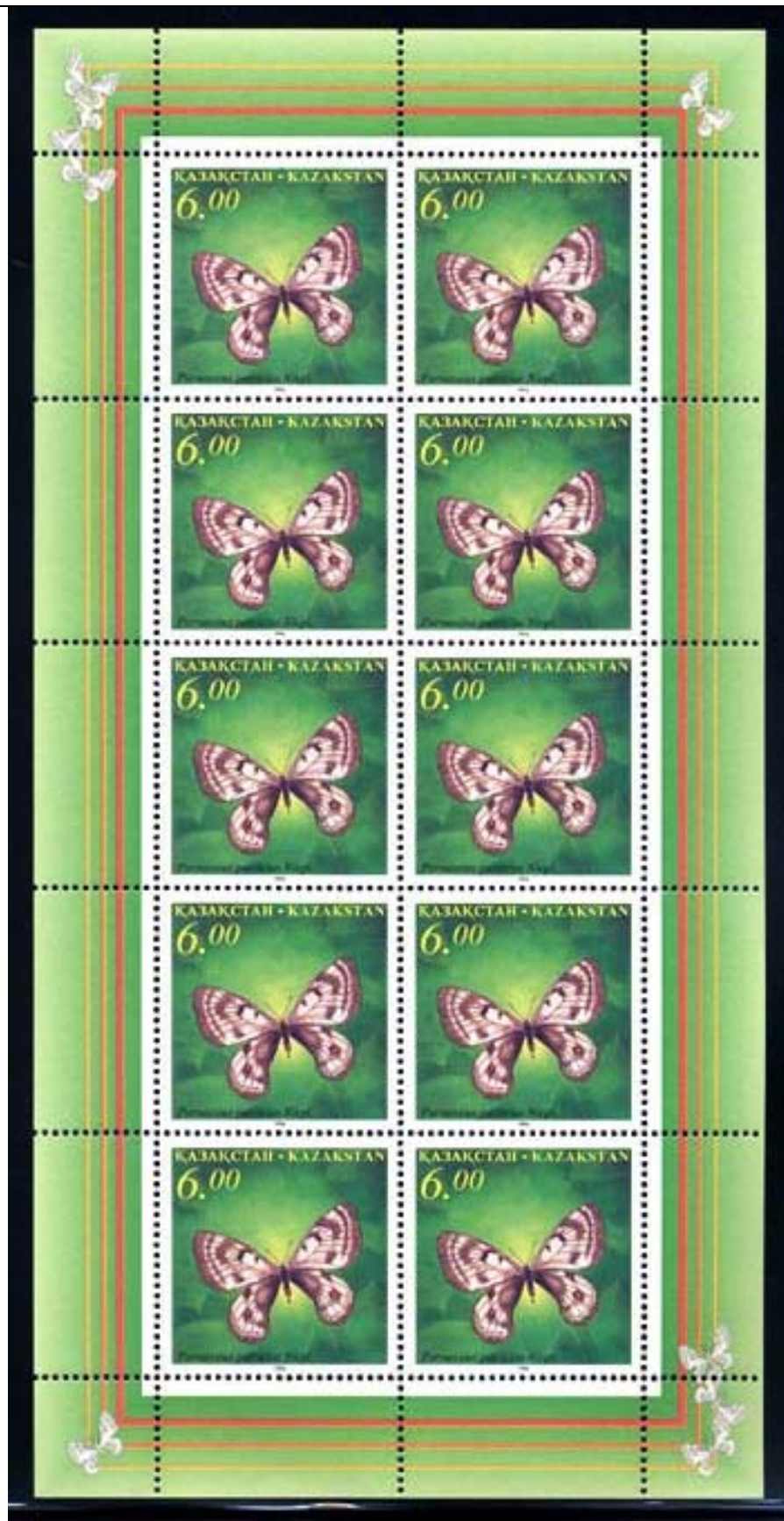
Lepidoptera : Papilionidae : Parnassius patricius .
