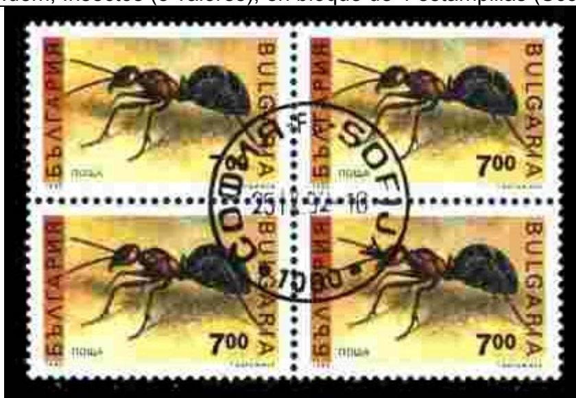
Hymenoptera : Formicidae
