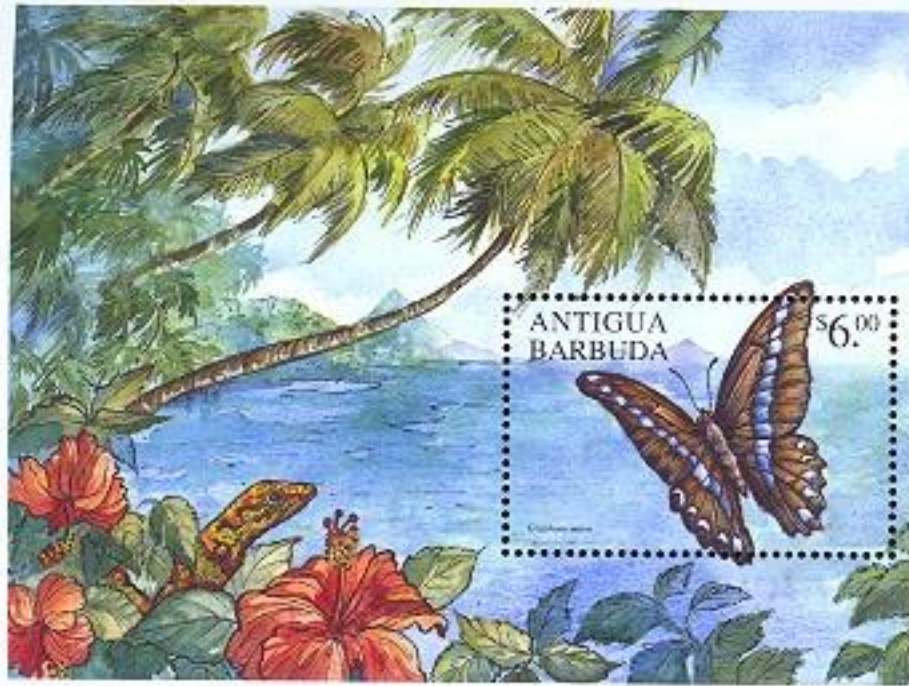
Lepidoptera : Papilionidae : Graphium milon .
