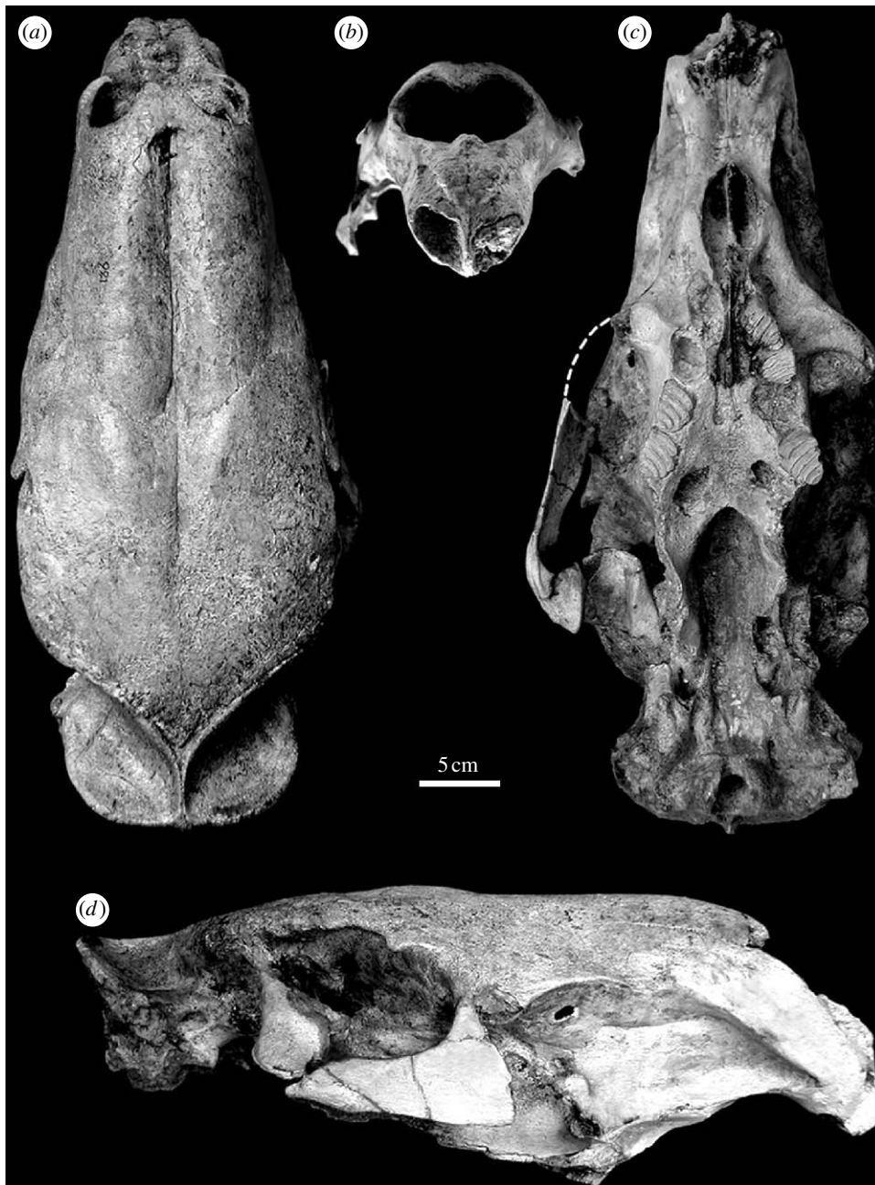
Figure 1. Skull of J. monesi sp. nov. (holotype, Museo Nacional de Historia Natural y Antropología MNHN 921) in (a) dorsal, (b) frontal, (c) ventral and (d) lateral views.
