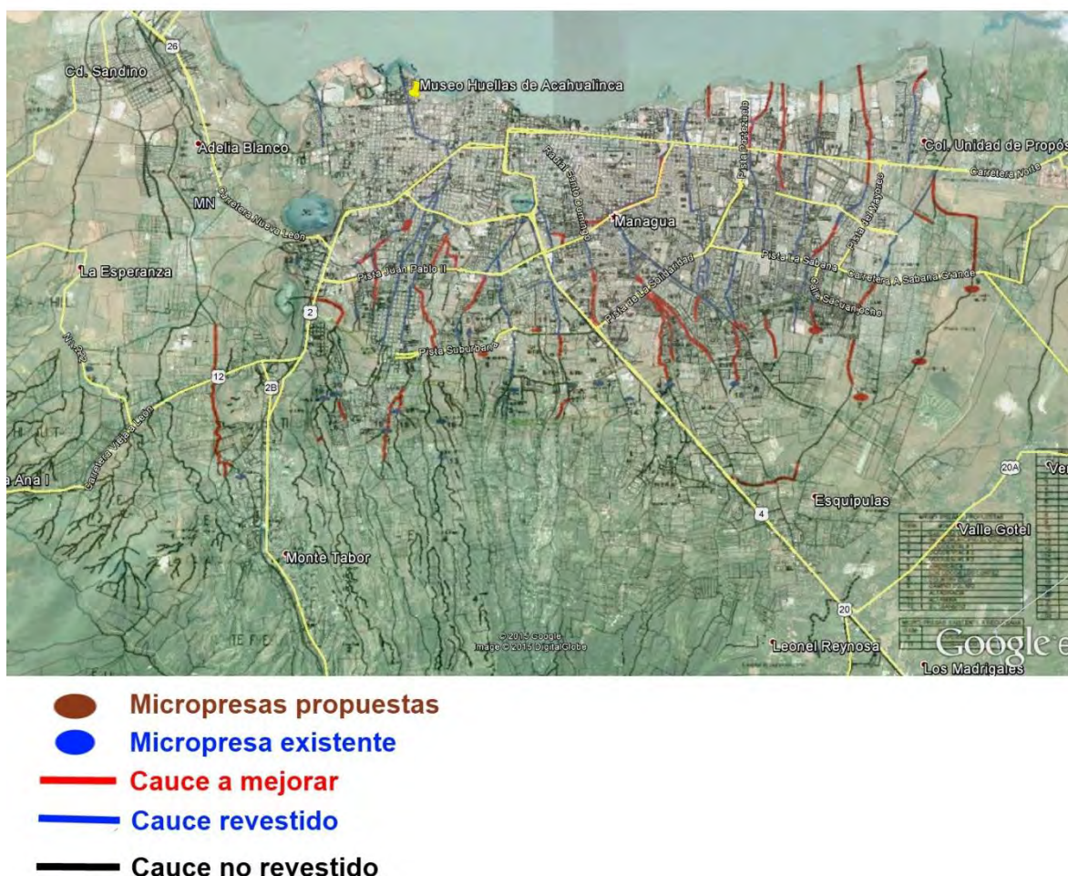
Figura 4. Red de acequias y cauces de la ciudad de Managua, modificado de; " Plano de la ciudad de Managua, ubicación de micropresas y cauces ", Dirección de Proyectos Municipales, Alcaldía de Managua.
