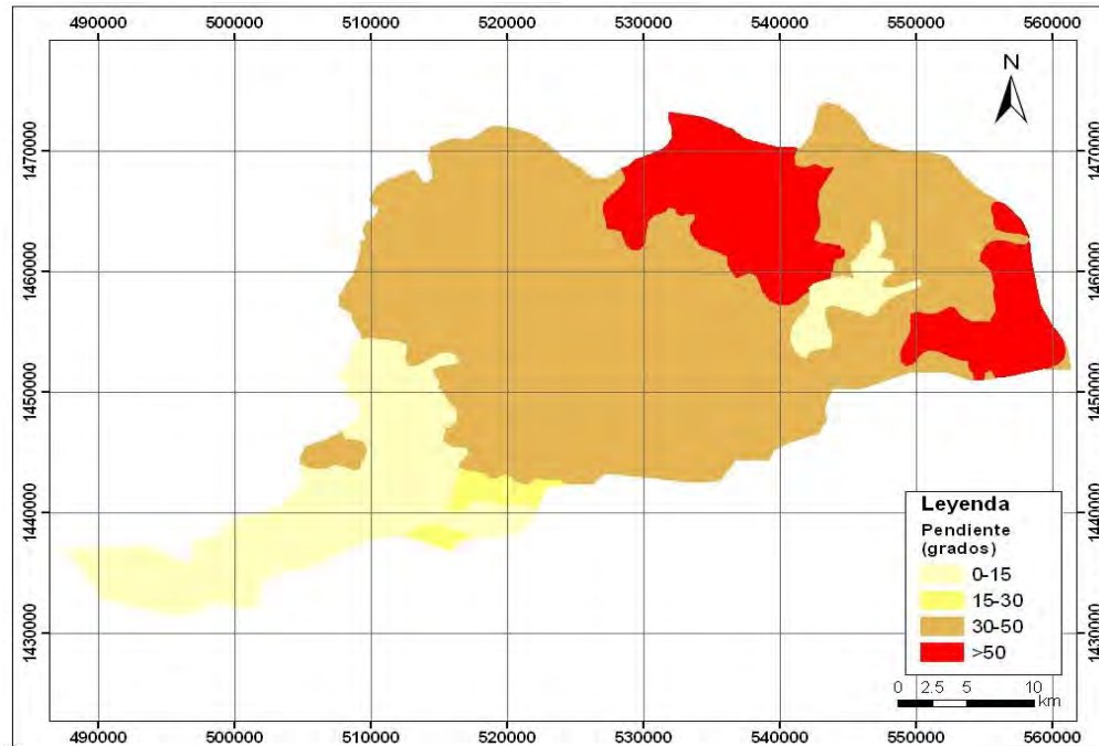
Figura 9. Distribución de Rangos de Pendiente. Cuenca N° 58
