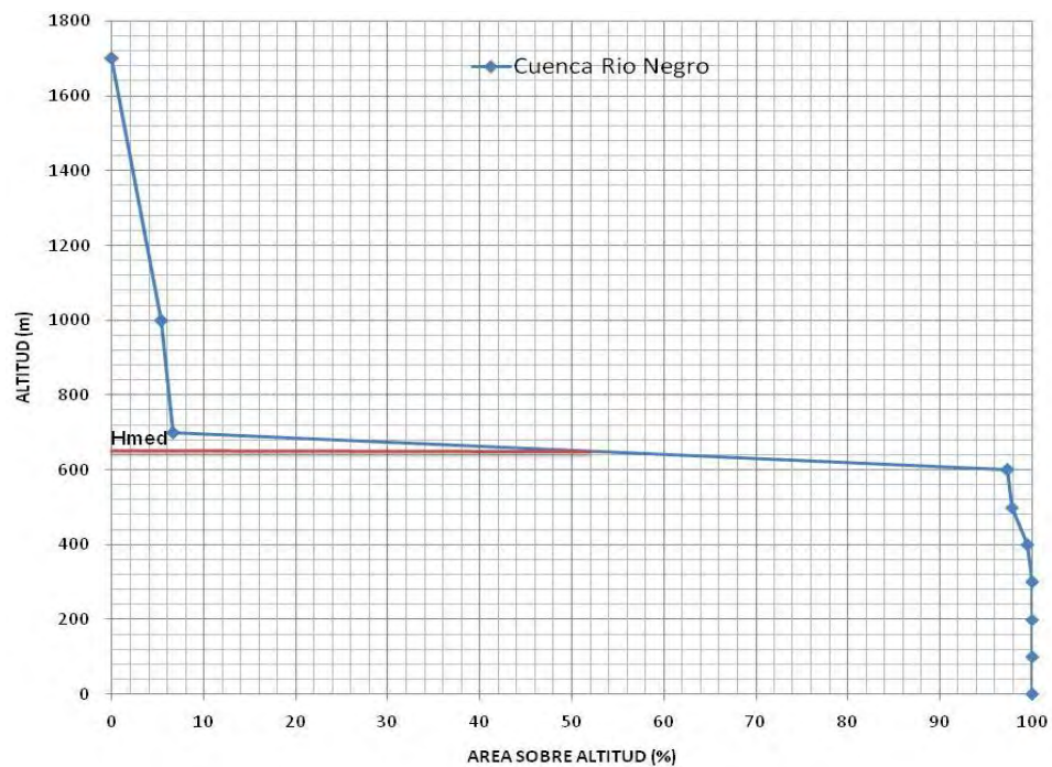
Figura 10. Curva Hipsométrica. Cuenca N° 58.
