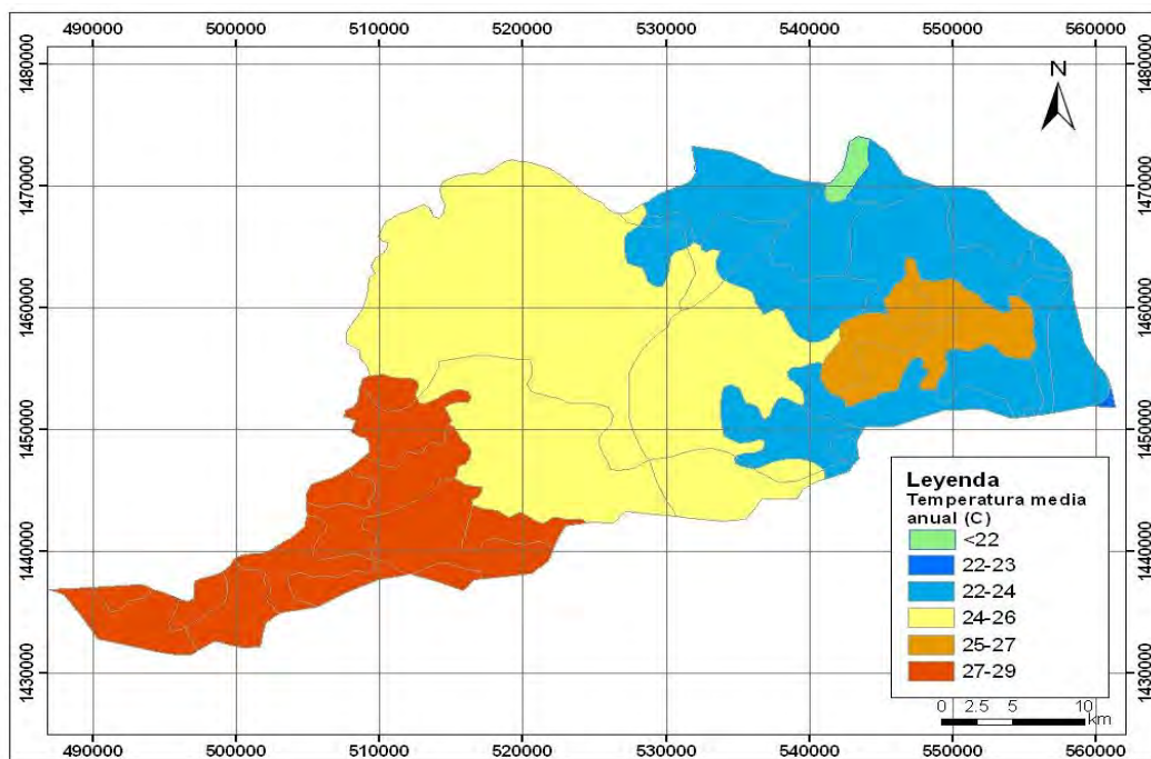
Figura 3. Distribución de los rangos de temperatura (°C) (Datos MAGFOR).Cuenca N° 58.
