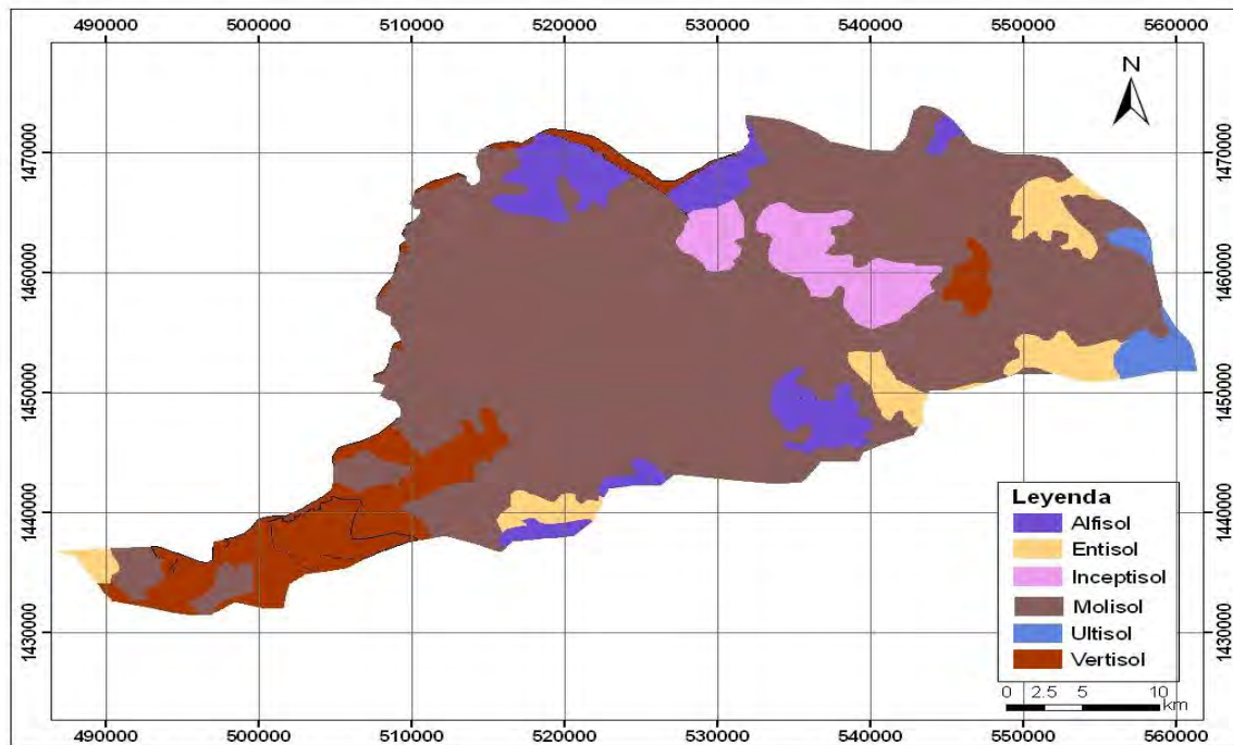
Figura 5. Orden de Suelos. Cuenca N° 58.
