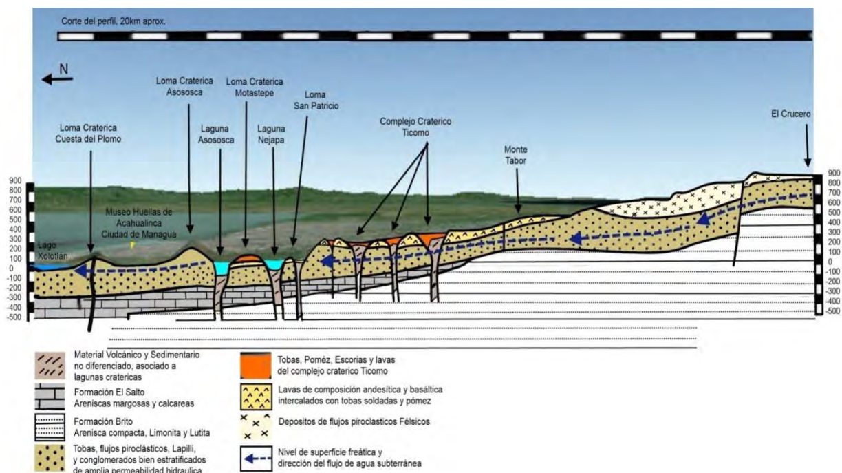
Figura 6. Perfil geológico generalizado representando el acuífero de la Cuenca sur del Lago de Managua y su flujo hidrogeológico freático. Modificado de Losilla et.al., 2001.
