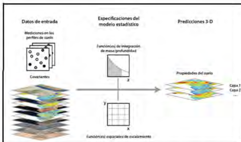
Figura 1. Representación esquemática del MDS. Las características del suelo en lugares conocidos se combinan con conjunto de datos asociados (covariantes) para, a través de modelos estadísticos, extrapolar las propiedades del suelo a zonas de las que no hay datos. (Fuente: Atlas de Suelos de América Latina y El Caribe).
