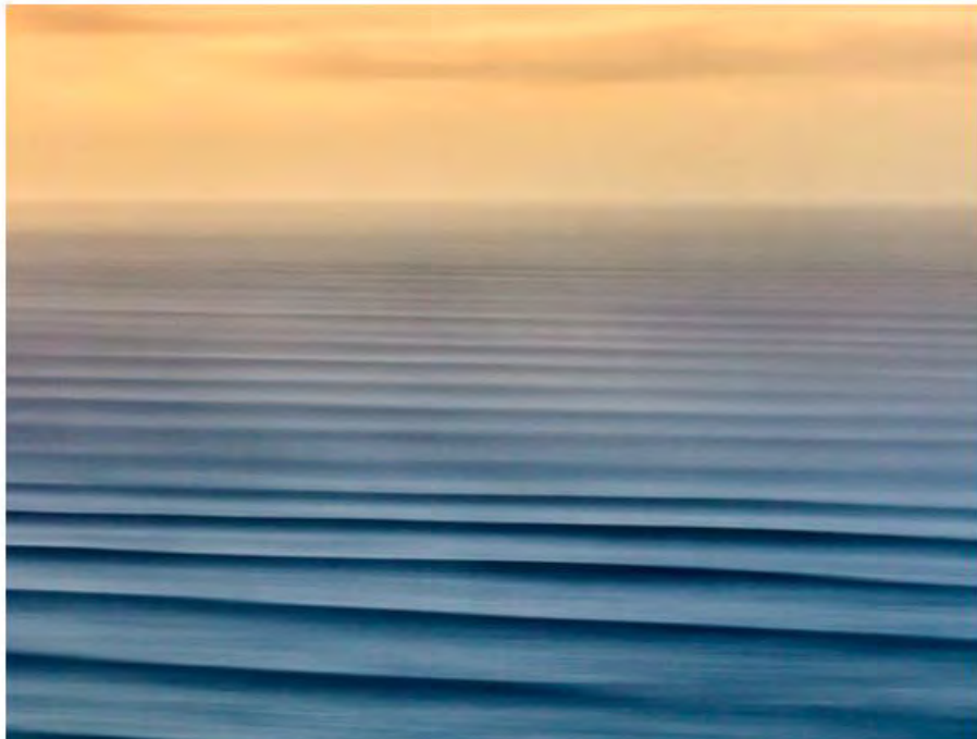
Fig. 2. Oleaje ordenado de mar de fondo.
