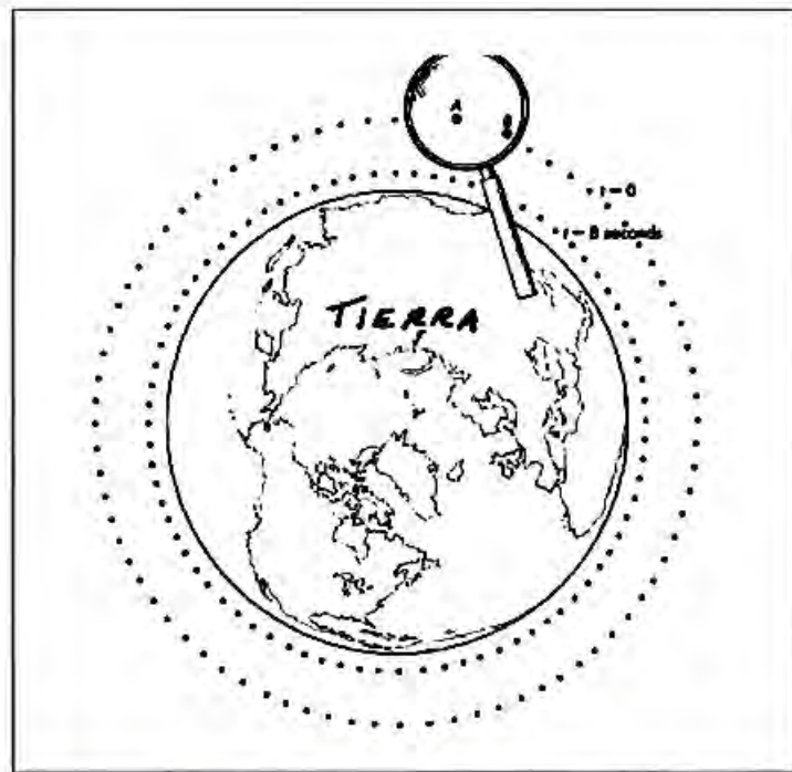
Figura 20. Efecto de reducción de volumen. Este efecto ocurre en proximidad a la superficie de la tierra. El efecto de reducción de volumen es mayor que el efecto de marea y totalmente domina. El efecto global manifestado en el conglomerado de marcos locales da la apariencia de una fuerza global de atracción hacia el centro de la tierra.
