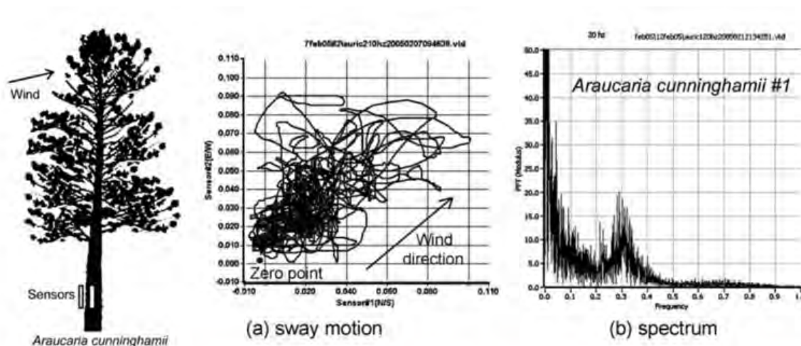
Movimiento de balanceo de Araucaria cunninghamii (velocidad del viento promedio de 12 m/seg) que muestra (a) complejo movimiento de oscilación del tronco del árbol (viento abajo desde el punto de registro) y (b) espectro que muestra la frecuencia de oscilación con pico único a 0,29 Hz.
