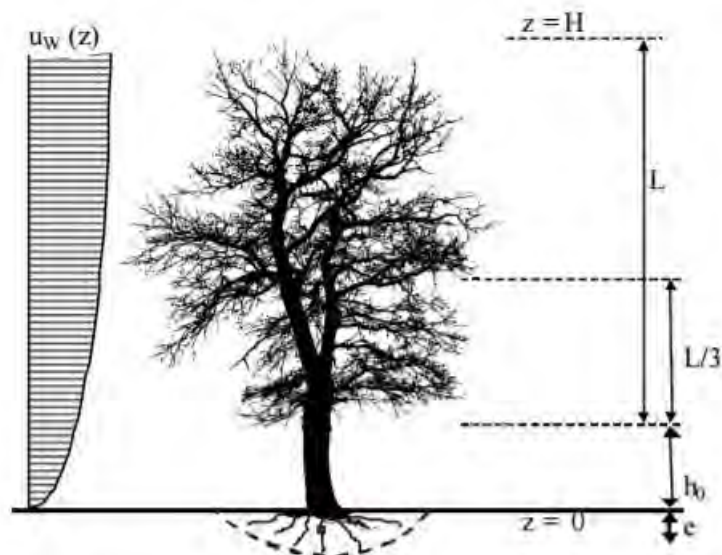
Presión dinámica sobre un árbol
